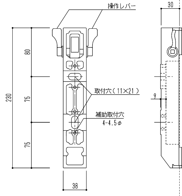
取付ブラケット詳細図
